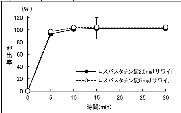
<50rpm:pH1.2>
