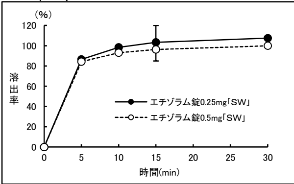
<50rpm: pH1.2>
