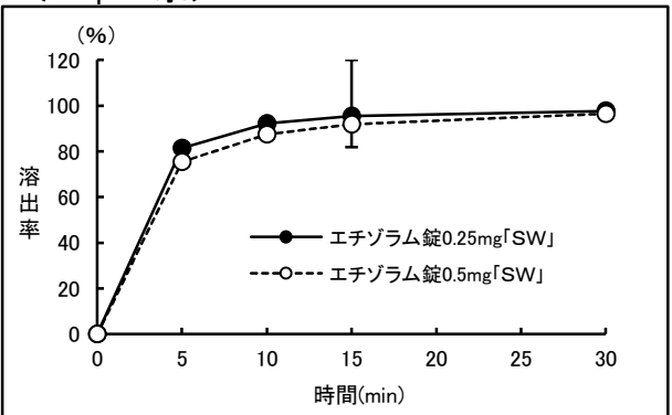
<50rpm: 水>
