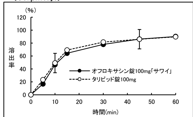
&lt;50rpm:水&gt;
