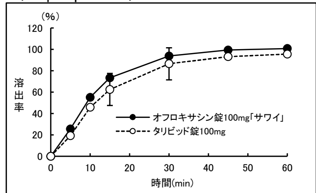
&lt;50rpm:pH4.0&gt;
